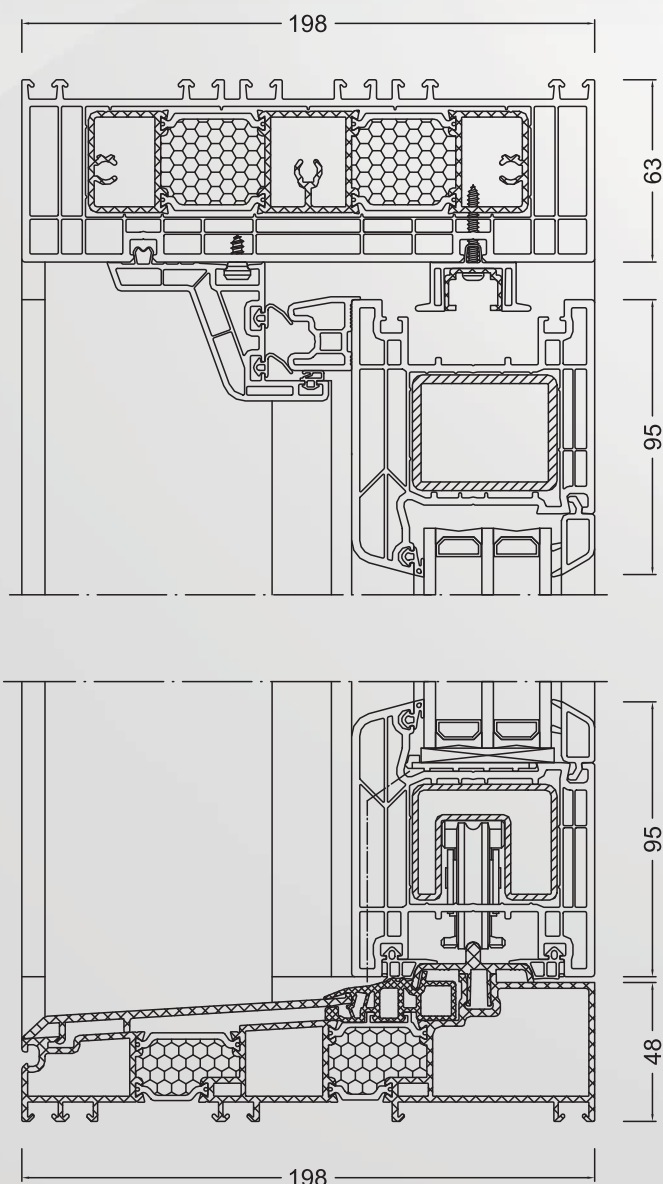
Vertikalschnitt:
