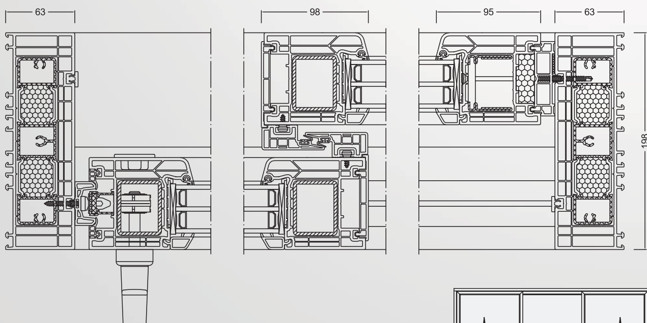
Horizontalschnitt:
